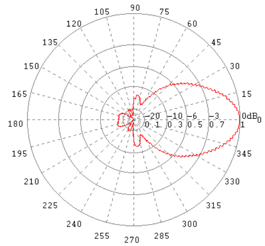
H-Ebene / H-Plane 800 MHz
